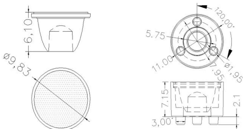
透镜外形尺寸 Len profile dimensions
